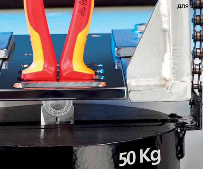
Проверка надежности соединения электроизолированных чехлов с ручками инструмента под нагрузкой 500 Н.
